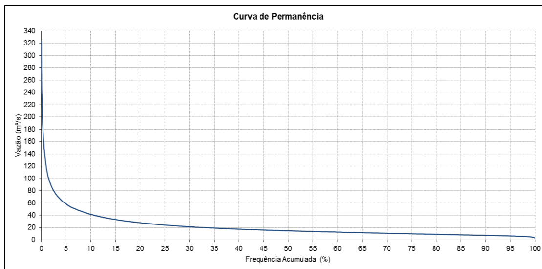
Figura 3-14 - Curva de permanência da estação Baixo Guandu.
