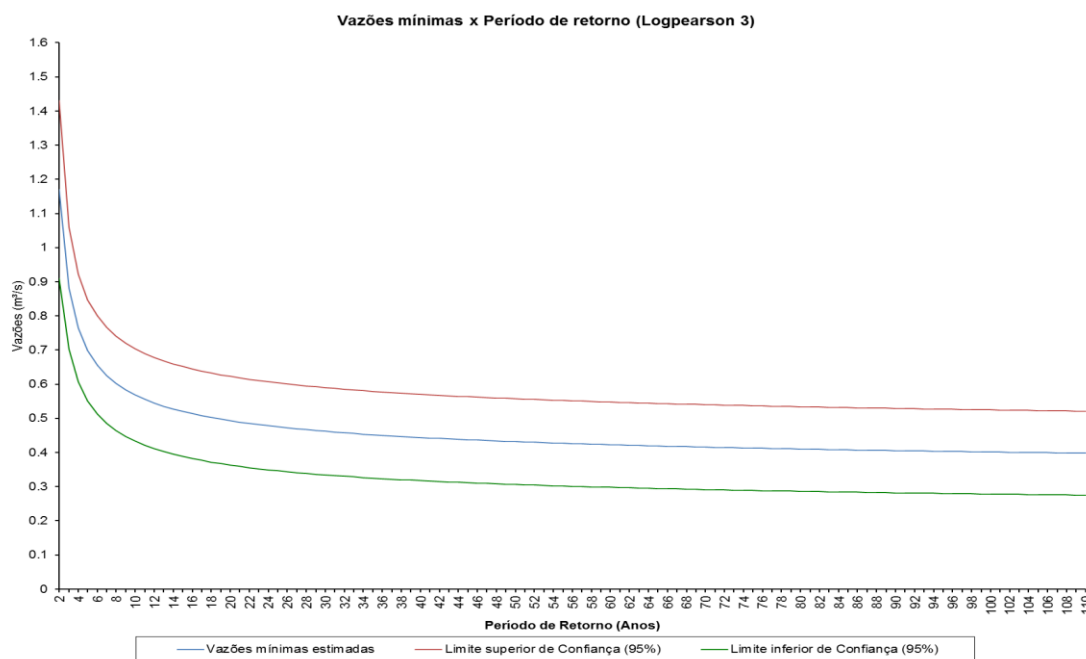
Figura 3-16 - Gráfico da vazão mínima associada a cada período de retorno estimado pela distribuição Log Pearson 3 para a estação Ponte do Pancas.
