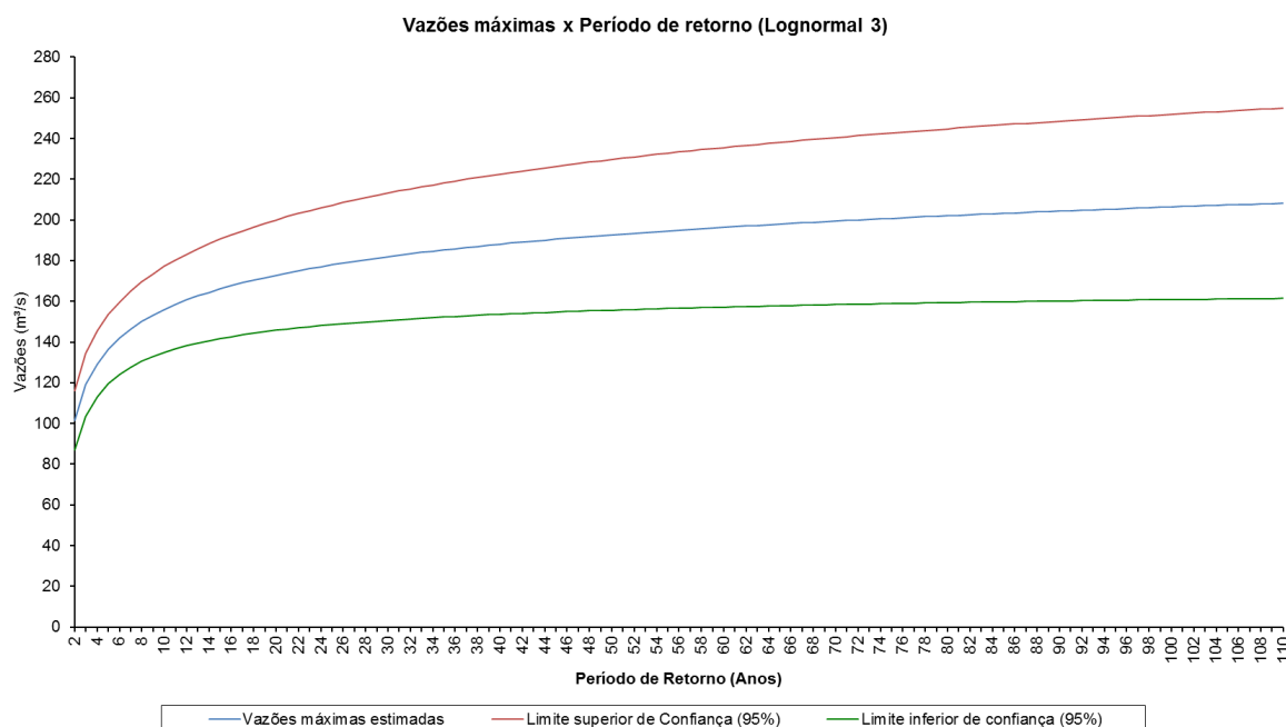
Figura 3-15 - Gráfico da vazão máxima associada a cada período de retorno estimado pela distribuição Lognormal3 para a estação Barra de São Gabriel.
