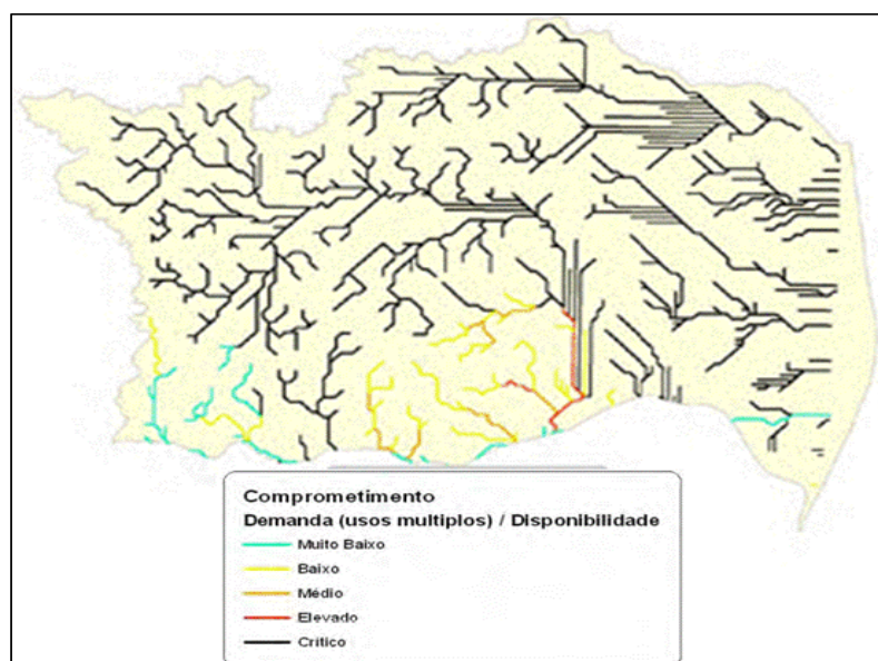
Figura 3-31 - Saldos hídricos para o cenário tendencial 2030 na UA São José, segundo a modelagem.
