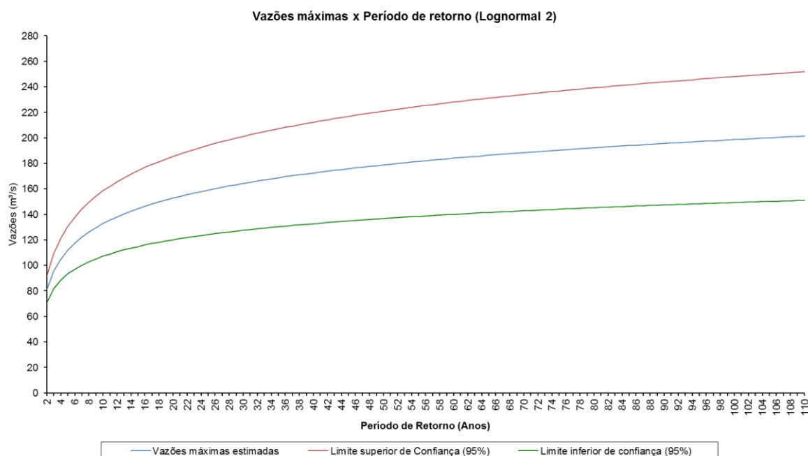
Figura 3-14 - Gráfico da vazão máxima associada a cada período de retorno estimado pela distribuição Lognormal2 para a estação Ponte do Pancas.
