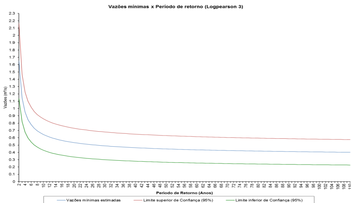
Figura 3-17 - Gráfico da vazão mínima associada a cada período de retorno estimado pela distribuição Log Pearson 3 para a estação Barra de São Gabriel.
